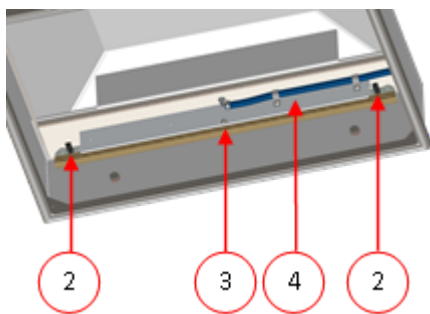
Figura 23: Extracción de la barra de sellado
