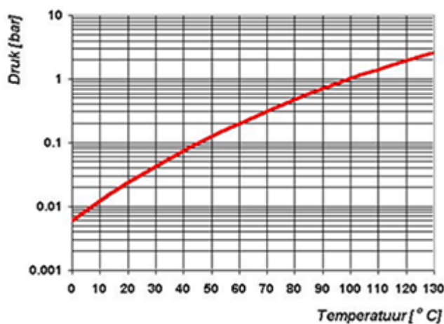
Figura 30: Curva de presión de vapor del agua
