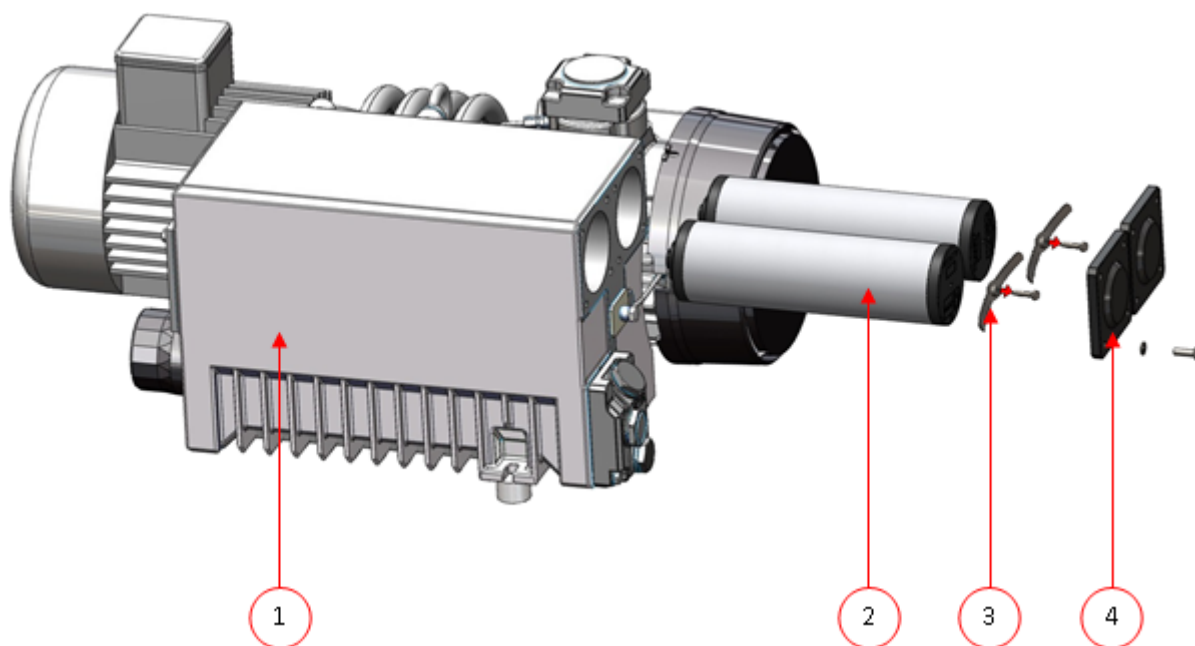
Figura 29: Sustitución del filtro de salida de aceite
