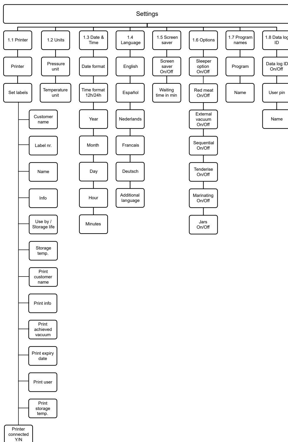
Figura 11: Descripción general del menú Ajustes
