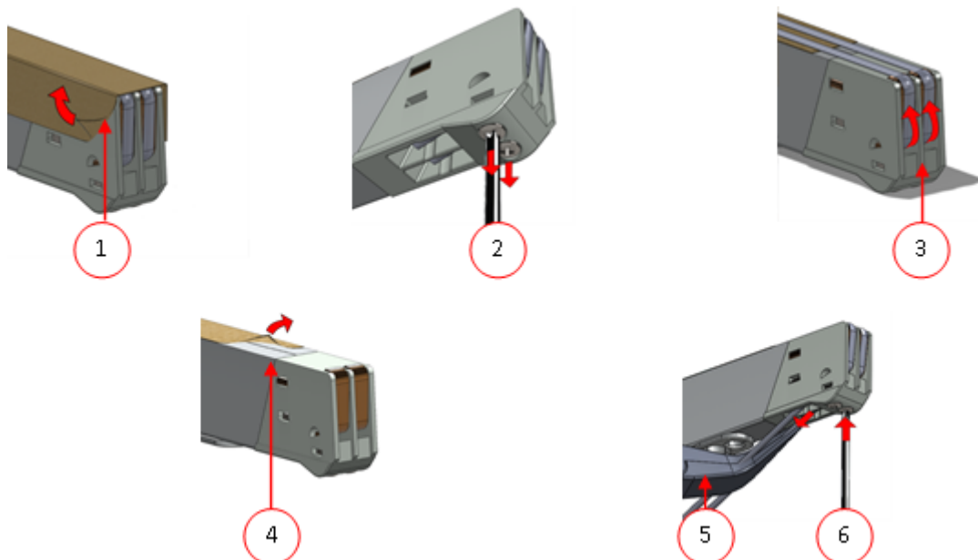
Figura 25: Sustitución del alambre de sellado
