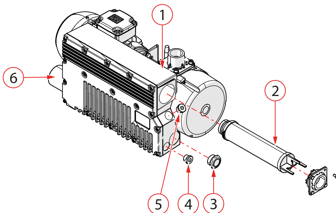
Figura 30: Descripción general de la bomba Becker
