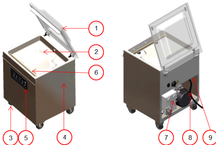
Figura 2: Descripción general de los componentes principales
