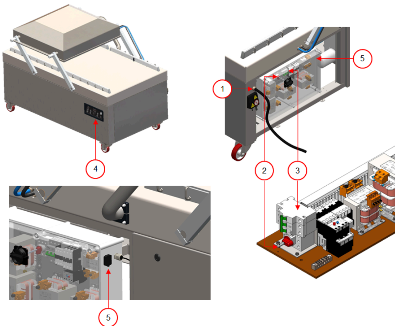
Figura 35: Descripción general de la instalación eléctrica, Falcon, Polar
