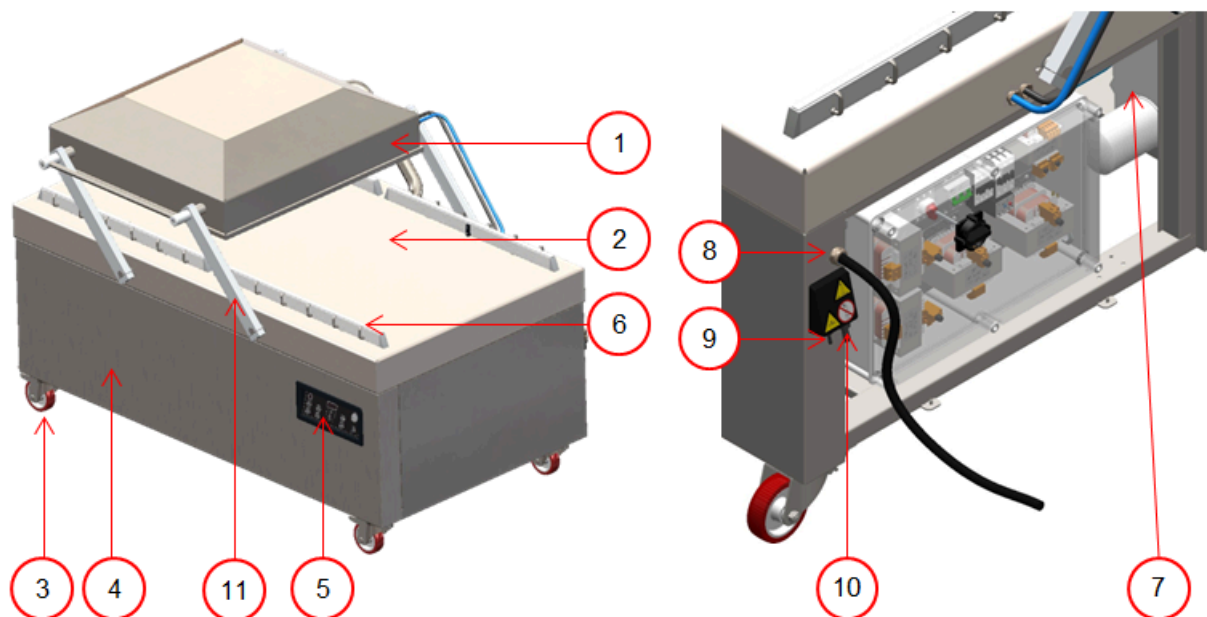
Figura 3: Descripción general de los componentes principales
