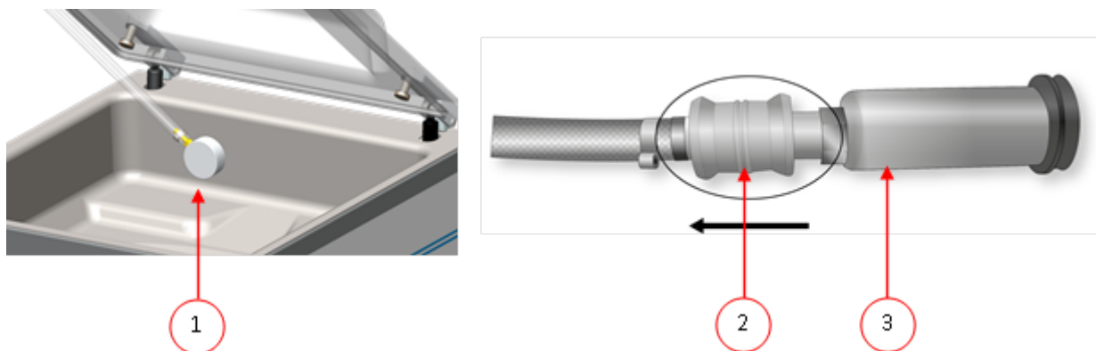
Figura 17: Juego de adaptador de vacío externo (ACS)
