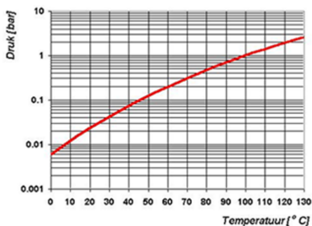
Figura 36: Curva de presión de vapor del agua
