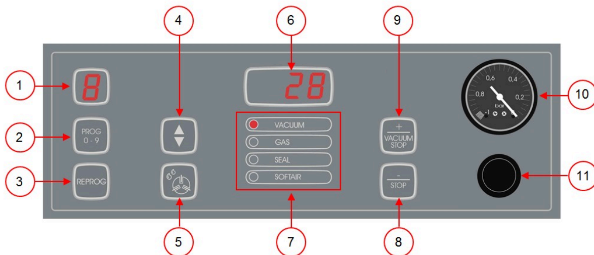
Figura 9: Panel de control del sistema de control de 10 programas
