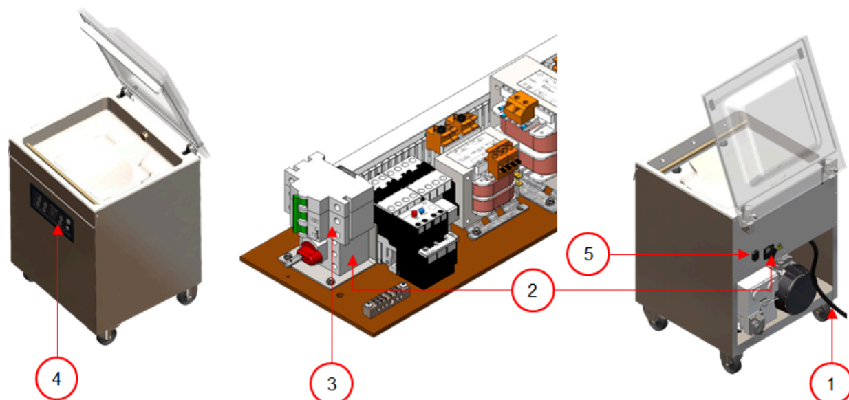
Figura 34: Descripción general de la instalación eléctrica, Marlin
