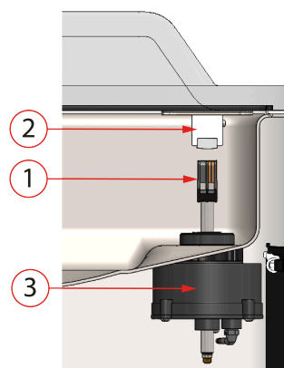
Figura 6: Descripción general del sistema de sellado (incluye el cilindro de sellado)
