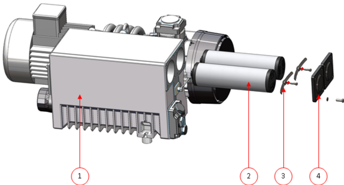
Figura 33: Sustitución del filtro de salida de aceite
