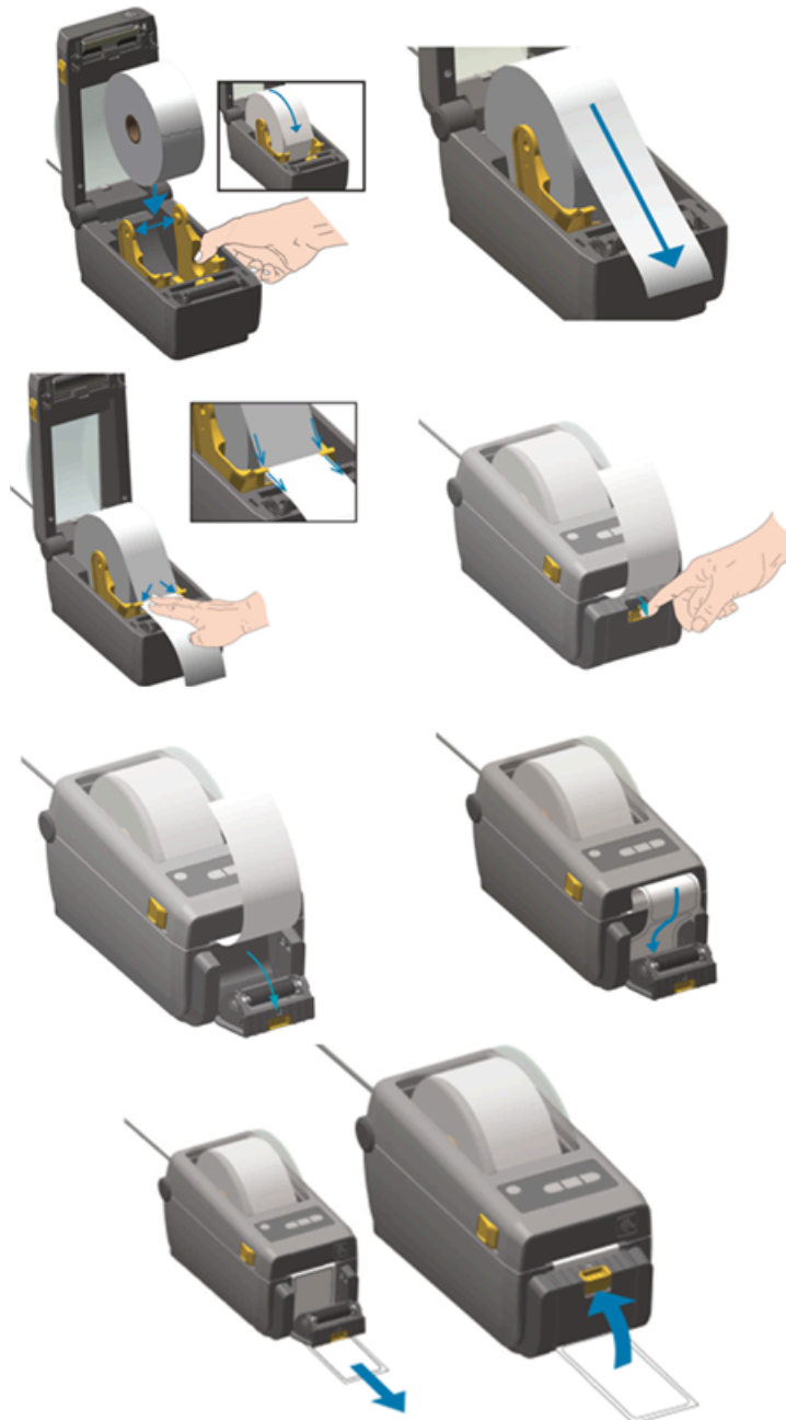
Figura 18: Sustitución del rollo de impresión
