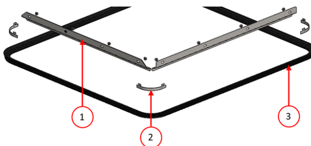
Figura 18: Sustitución de la junta de la tapa
