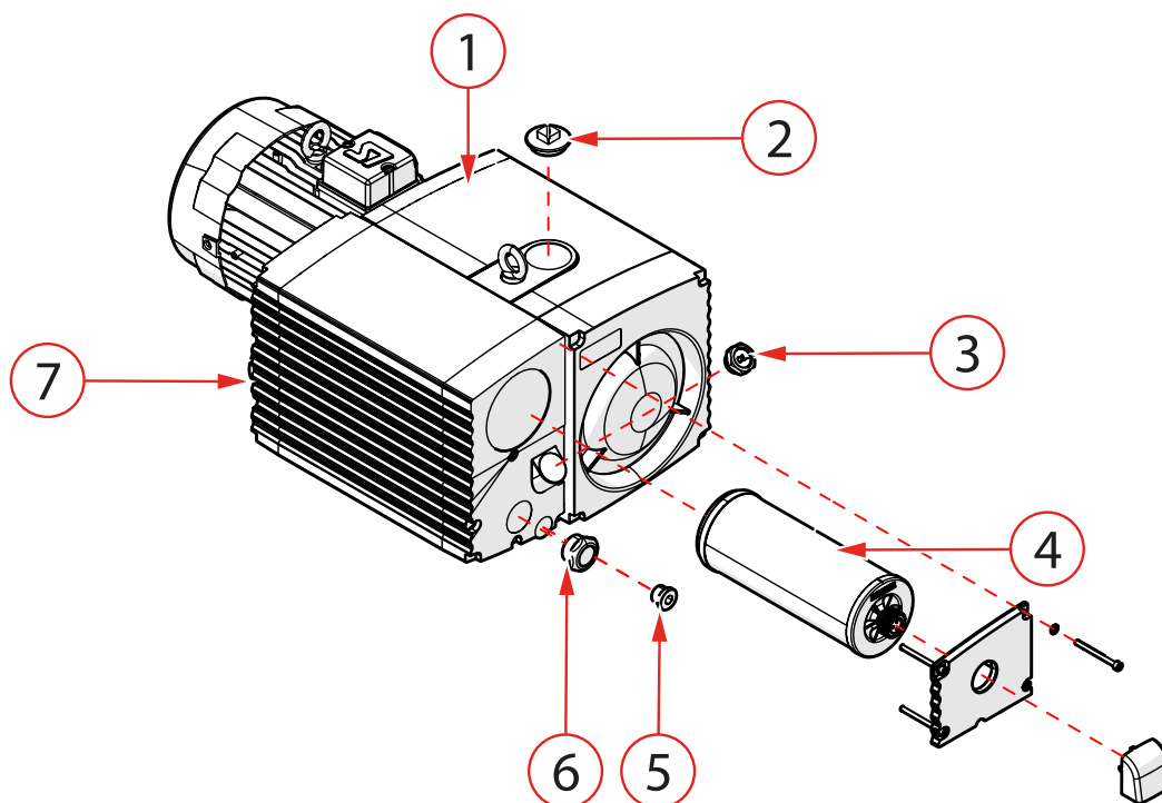
Figura 20: Descripción general de la bomba Becker
