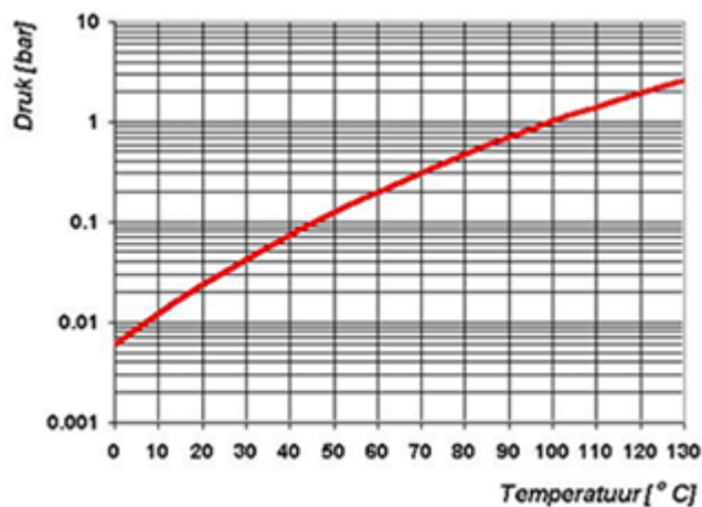
Figura 23: Curva de presión de vapor del agua
