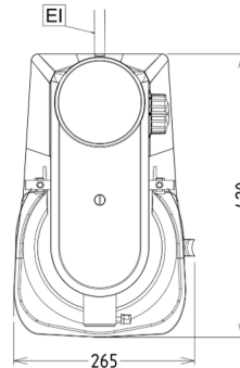
Boven aanzicht
