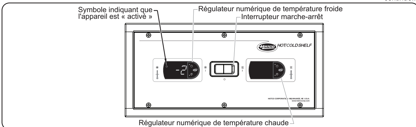
Boîtier de commande de la plaque chauffante/réfrigérante (en mode FROID)
