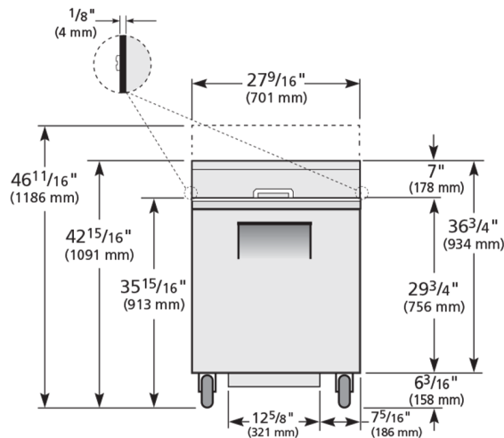
ELEVATION
